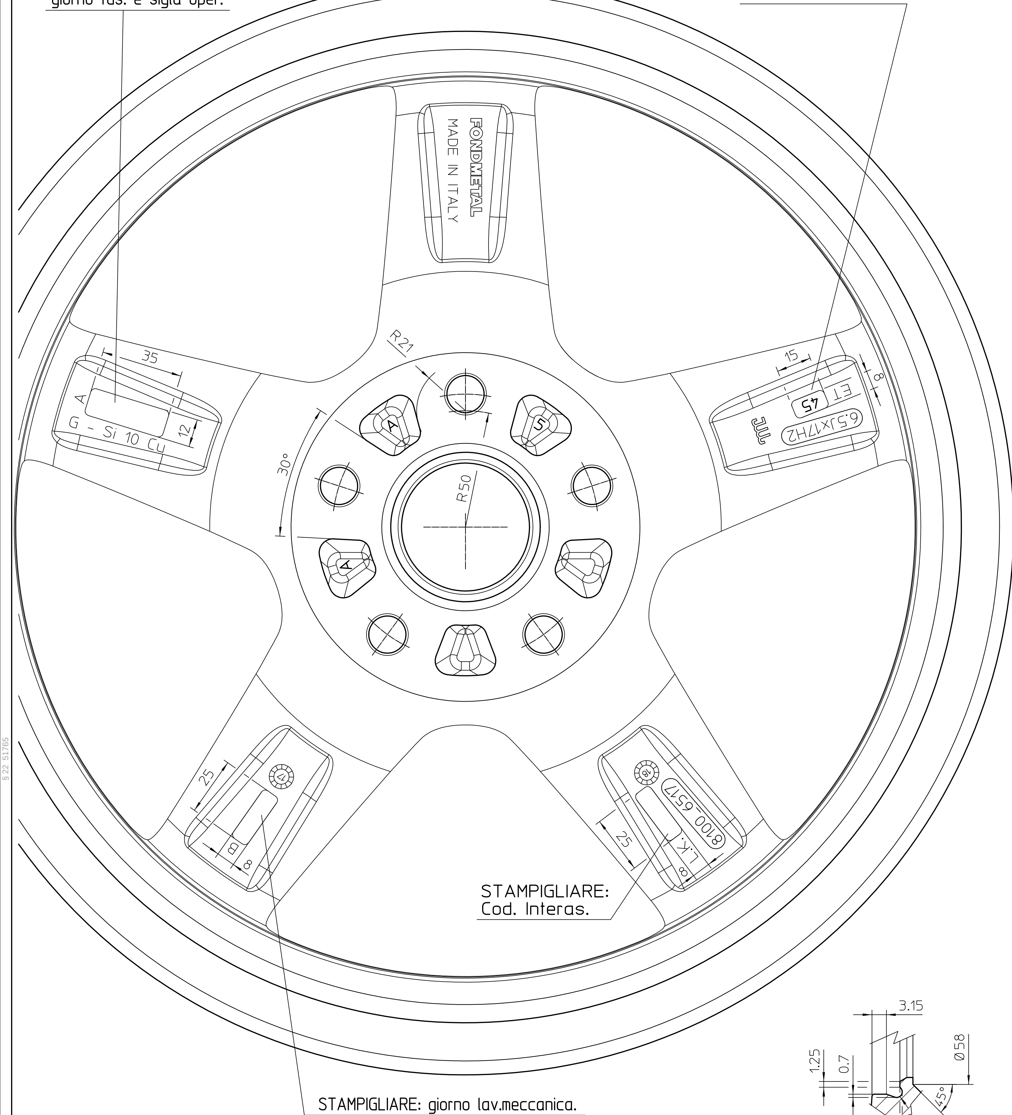
DETAIL Massstab 2:1
