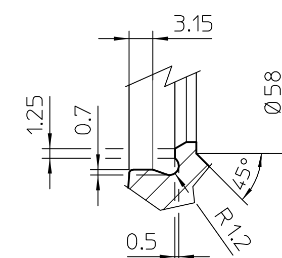
DETAIL Massstab 2:1
