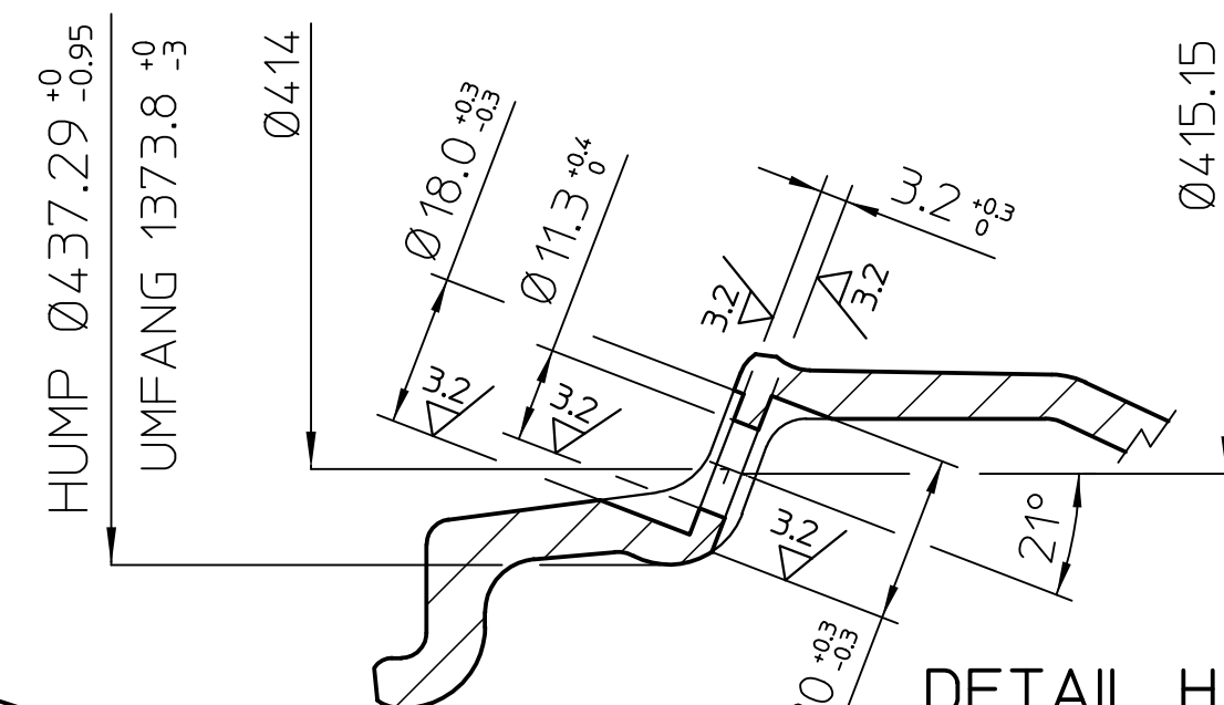
DETAIL H Massstab 1:1
