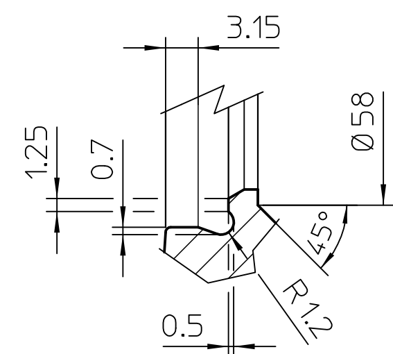
DETAIL Massstab 2:1
